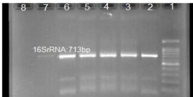
شکل ۲. نتیجه آزمون PCR برای جنس مایکوپلازما - ژن 16SrRNA: ردیف ۱: Lader 100 bp، ردیف ۲: کنترل مثبت (سویه استاندارد مایکوپلازما پنومونیه ATCC: 29342)، ردیف ۳ تا ۷: نمونه هایی از جنس مایکوپلازما جدا شده از بیماران، ردیف ۸: کنترل منفی می باشند.
