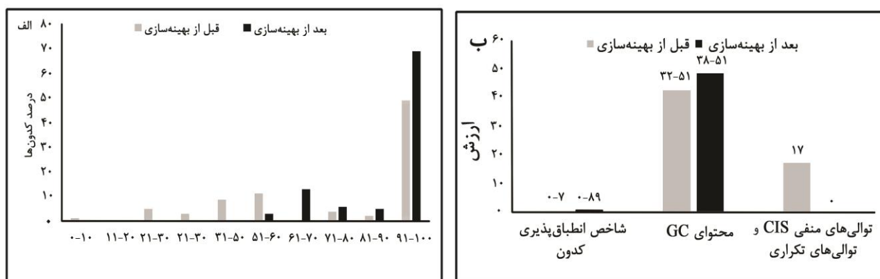
شکل ۴. بررسی توزیع فراوانی کدون‌ها بر اساس میزان تأثیر بر بیان پروتئین (الف) شاخص سازگاری کدون، درصد GC و توالی‌های منفی و تکراری مؤثر در بیان پروتئین (ب). در نمودار الف، محور عمودی نشان دهنده درصد کدون‌های پروتئین می باشد و محور افقی نشانگر دسته‌بندی و ارزش گذاری کدون‌ها بر اساس میزان تأثیر بر بیان پروتئین، و ارزش زیر ۳۰ به معنی تأثیر منفی بر بیان پروتئین است. در نمودار ب، بهبود شاخص‌های مؤثر بر بیان پروتئین ارائه شده است. همانطور که در نمودار ب دیده می شود شاخص انطباق پذیری کدون به ۸۹٪ ارتقاء یافته و توالی‌های منفی و تکراری مؤثر بر بیان پروتئین نیز حذف گردیده است.
