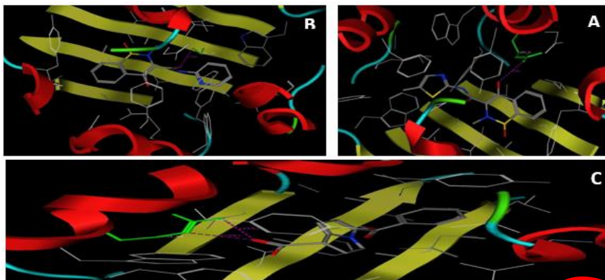
شکل ۲: باندهای هیدروژنی LasR (A) ملوکسیکام، (B) پیروکسیکام، (C) کتورولاک
