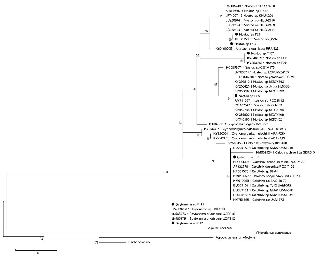
شکل ۲. شکل درخت فیلوژنتیک را نشان می دهد. مقیاس نشان داده شده در شکل، نشان دهنده ۰/۰۵ جهش به ازای هر نوکلئوتید است. نمونه های مورد مطالعه با دایره توپور نشان داده شده است.
