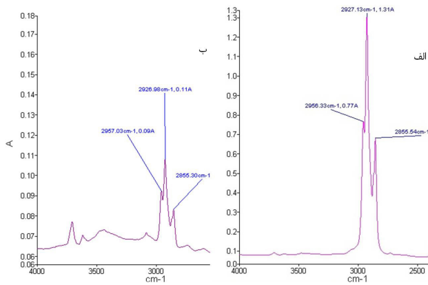
تصویر شماری ۴: طیف جذبی FTIR برای Phaeosphaeria spp. UTMC 5003 : الف: طیف جذبی نمونه شاهد و ب: طیف جذبی در محیط کشت PDB همراه با ۱ درصد نفت. کاهش ۹۰ درصدی در طول موج 2960\text{ cm}^{-1} و 2930\text{ cm}^{-1} در نمونه تیمار شده نسبت به نمونه‌ی شاهد قابل مشاهده است
